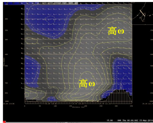
圖 5：2014 年 05 月 15 日 0600UTC \omega (-ubar/s) 場：成熟階段的飆線，在中層以上有另一 \omega 高值區，診斷分析是由上升空氣帶著低層入流區的動量上升達對流層中上層而致。此說明深對流的發展與大氣中上層的 \omega 高值出現有明顯的關係。
