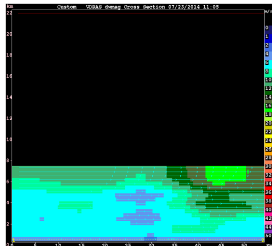
圖 6：2014 年 7 月 23 日 1105 UTC 橫跨飆線之 VDRAS dwmag(垂直風切風速量) 2D 垂直剖面及徑向風流線圖，顯示在飆線右側上空有強垂直風切，風速達 18m/s。
