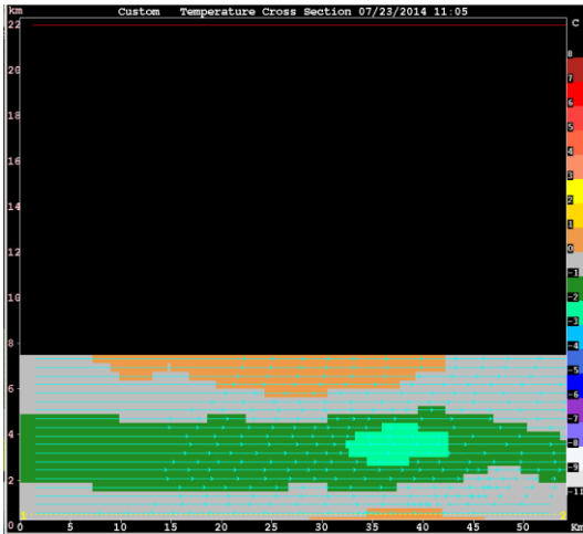
圖 7：2014 年 7 月 23 日 1105 UTC 橫跨颶線之 Temperature 2D 垂直剖面及徑向風流線圖，顯示在颶線 3 至 4km 上空有冷空氣，這是中層的后部內流 (rear inflow) 注入冷空氣與下衝氣流(down draft)的例證。
